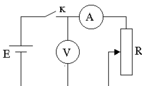
7 – rasm. EYUK va ichki qarshilikni aniqlash sxemasi.
