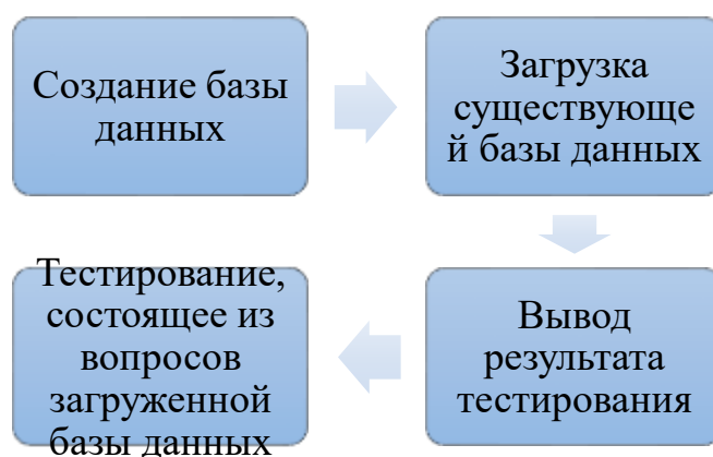
Рисунок 1. Тестирующей программы.
