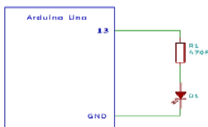
2-rasm. Arduino Uno qurilmasiga LEDni ulash printsiplial elektr sxemasi
